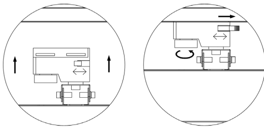
Рисунок 10. Крепление на шинопроводе.
