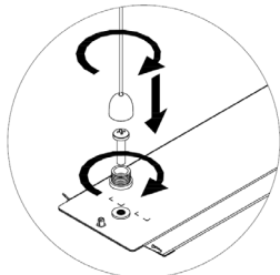
Рисунок 7 – Установка подвесным способом .
