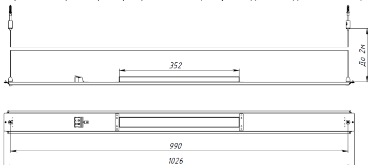
Рисунок 5 – Вариант установки тросовых подвесов при комплектации с креплением подвес 08881/08882 (на примере Liner Basic 1026x66x25).
