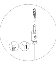
Рисунок 7 – Установка подвесным способом .
