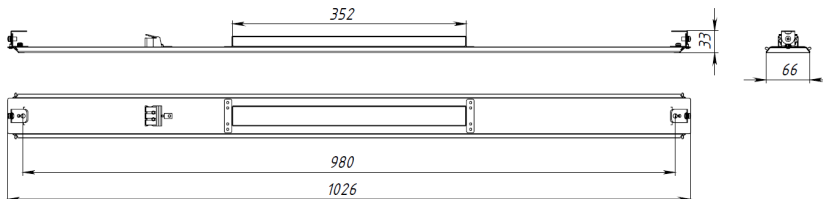
Рисунок 4 - Габаритные размеры при комплектации с уголок для накладного монтажа (на примере Liner Basic 1026x66x25).
