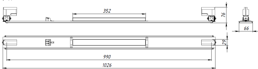
Рисунок 2 - Габаритные размеры при комплектации с креплением для шинпровода (на примере Liner Basic 1026x66x25).
